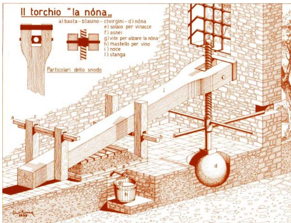
Fig. 69. Disegno di Lino Rizza raffigurante un torchio a leva di Esine, simile a quello di Piazzola
